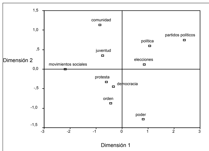
Figura 3 Escalamiento multidimensional
